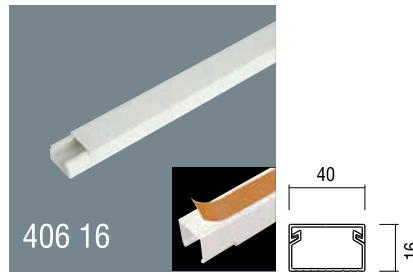
40x16 PVC Yapışkan Bantlı Kablo Kanalı Kapaklı Satılır Ambalaj: 60m / 30 Boy 40x16 Self Adhesive PVC Cable Trunking With cover Packaging: 60m / 30 Pcs
