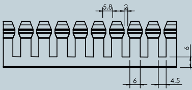
Yükseklığı 30/40mm olan kanalların delik ölçüleri Overall Height 30/40mm
