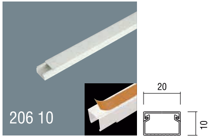
20x10 PVC Yapışkan Bantlı Kablo Kanalı Kapaklı Satılır Ambalaj: 260m / 130 Boy 20x10 Self Adhesive PVC Cable Trunking With cover Packaging: 260m / 130 Pcs
