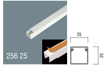
25x25 PVC Yapışkan Bantlı Kablo Kanalı Kapaklı Satılır Ambalaj: 80m / 40 Boy 25x25 Self Adhesive PVC Cable Trunking With cover Packaging: 80m / 40 Pcs
