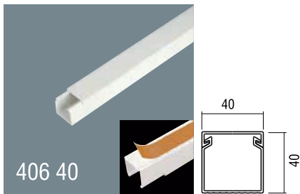
40x40 PVC Yapışkan Bantlı Kablo Kanalı Kapaklı Satılır Ambalaj: 48m / 24 Boy 40x40 Self Adhesive PVC Cable Trunking With cover Packaging: 48m / 24 Pcs
