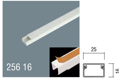
25x16 PVC Yapışkan Bantlı Kablo Kanalı Kapaklı Satılır Ambalaj: 128m / 64 Boy 25x16 Self Adhesive PVC Cable Trunking With cover Packaging: 128m / 64 Pcs
