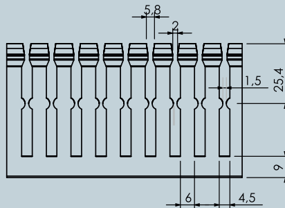
Taban genişliği 80mm olan kanalların delik ölçüleri
