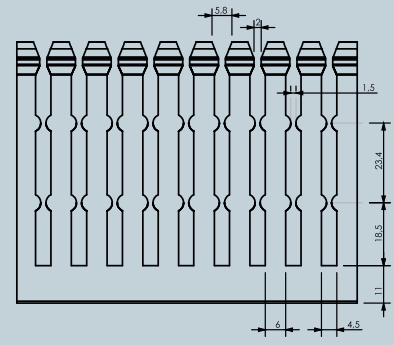
Taban genişliği 80mm olan kanalların delik ölçüleri
