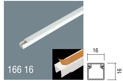
16x16 PVC Yapışkan Bantlı Kablo Kanalı Kapaklı Satılır Ambalaj: 192m / 96 Boy 16x16 Self Adhesive PVC Cable Trunking With cover Packaging: 192m / 96 Pcs
