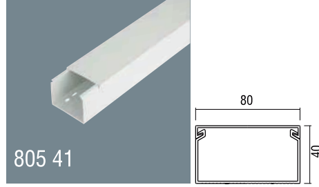
80x40 PVC Kablo Kanalı Kapaklı Satılır Ambalaj: 28m / 14 Boy 80x40 PVC Cable Trunking Complete with cover Packaging: 28m / 14 Pcs
