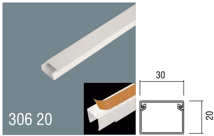
30x20 PVC Yapışkan Bantlı Kablo Kanalı Kapaklı Satılır Ambalaj: 84m / 42 Boy 30x20 Self Adhesive PVC Cable Trunking With cover Packaging: 84m / 42 Pcs
