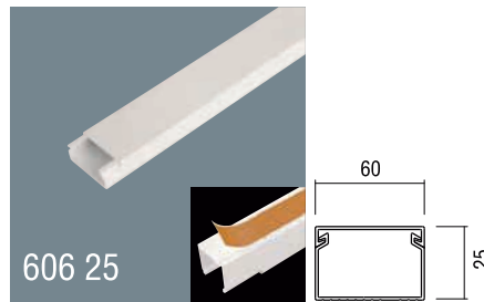
60x25 PVC Yapışkan Bantlı Kablo Kanalı Kapaklı Satılır Ambalaj: 48m / 24 Boy 60x25 Self Adhesive PVC Cable Trunking With cover Packaging: 48m / 18 Pcs
