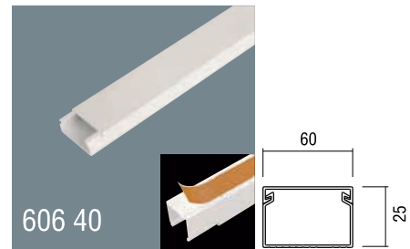
60x40 PVC Yapışkan Bantlı Kablo Kanalı Kapaklı Satılır Ambalaj: 36m / 18 Boy 60x40 Self Adhesive PVC Cable Trunking With cover Packaging: 36m / 18 Pcs
