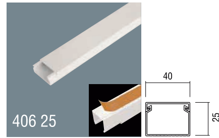
40x25 PVC Yapışkan Bantlı Kablo Kanalı Kapaklı Satılır Ambalaj: 50m / 25 Boy 40x25 Self Adhesive PVC Cable Trunking With cover Packaging: 50m / 25 Pcs
