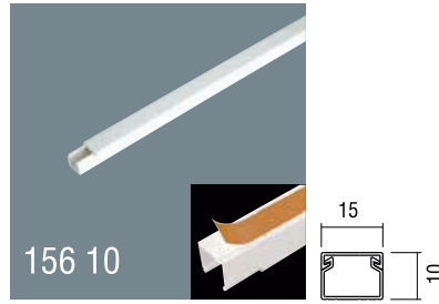
15x10 PVC Yapışkan Bantlı Kablo Kanalı Kapaklı Satılır Ambalaj: 364m / 182 Boy 15x10 Self Adhesive PVC Cable Trunking With cover Packaging: 364m / 182 Pcs
